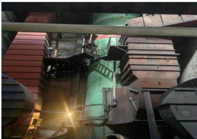
现有湿式脱硫除尘器
