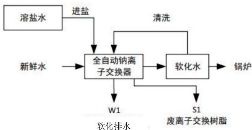
图 2-5 软水制备工艺流程及产污环节图
