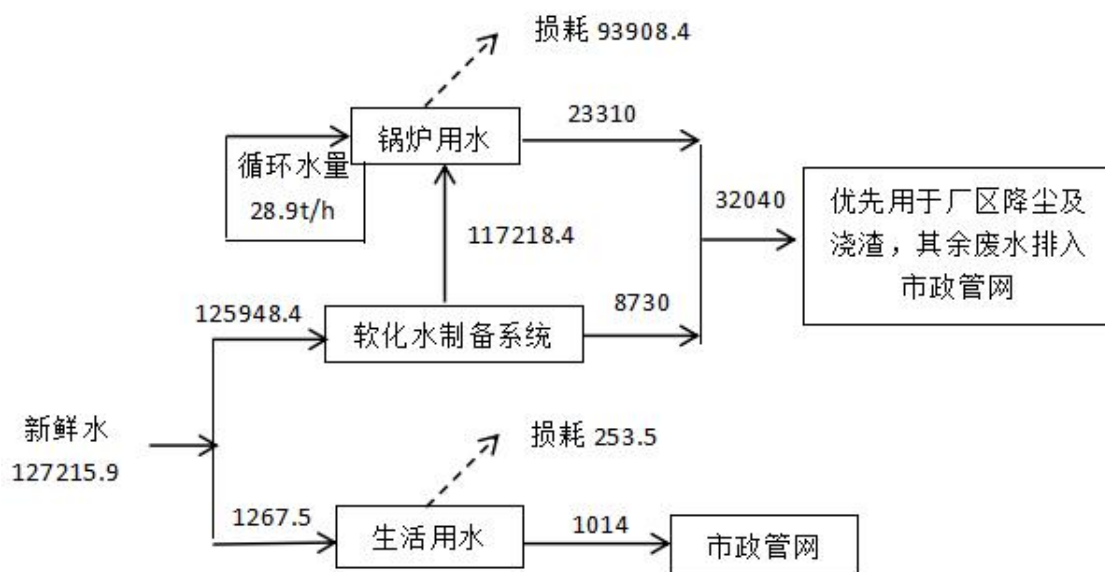
图 2-2 技术改造后全厂水平衡图 单位: \text{m}^3/\text{a}
