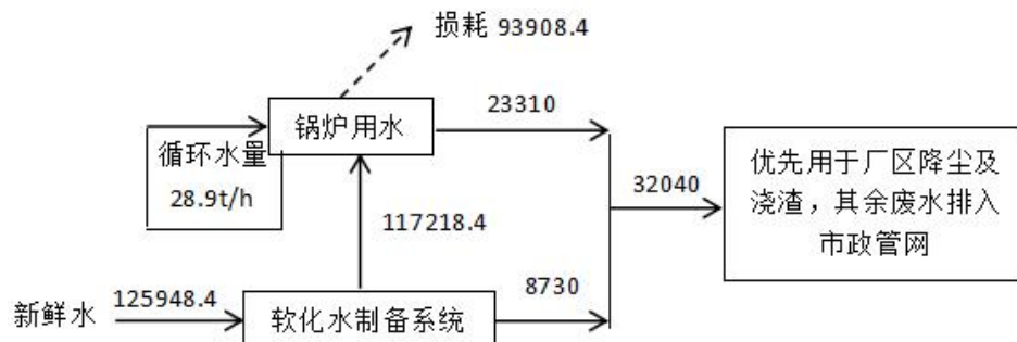
图 2-1 本项目水平衡图 单位：m³/a
